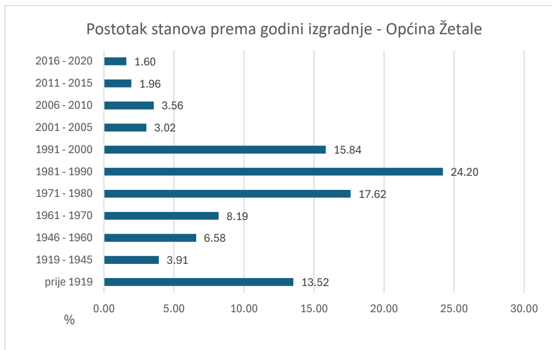
Graf 132: Postotak stanova prema godini izgradnje – Općina Žetale
