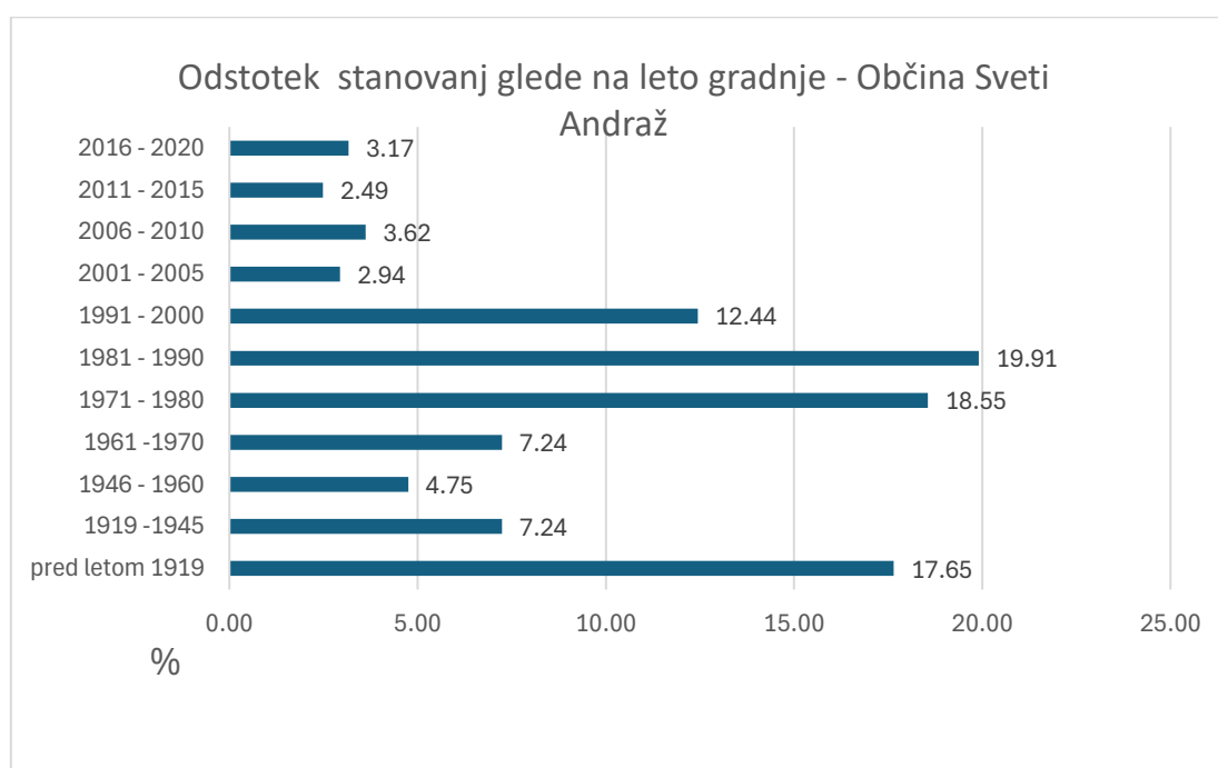
Graf 292: Odstotek stanovanj glede na leto gradnje – Občina Sveti Andraž v Slov. goricah
