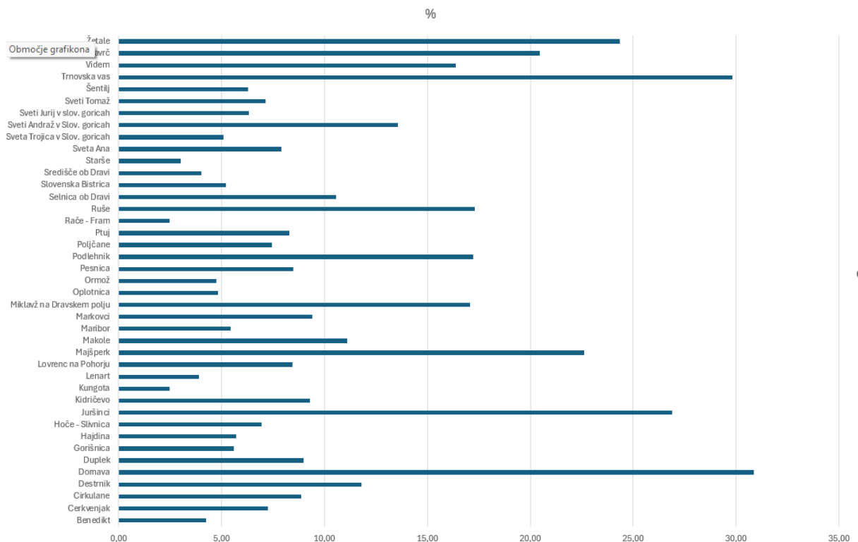
Graf 5: Udio energetskega siromaštva po opčinama
