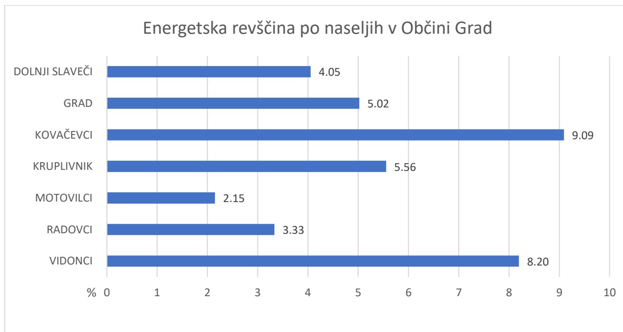
Graf 211: Energetska revščina v odstotkih po naseljih v Občini Grad
