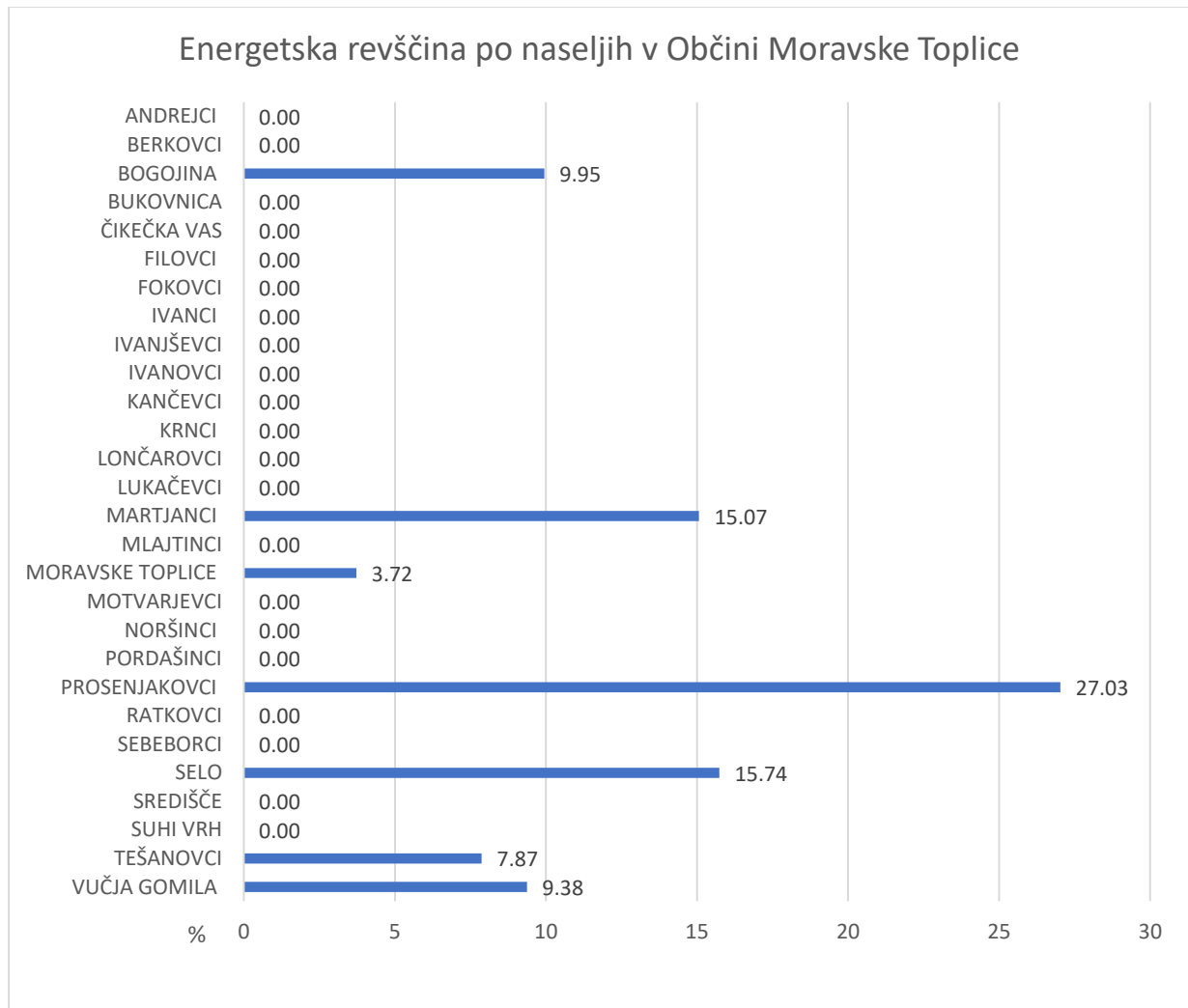
Graf 218: Energetska revščina v odstotkih po naseljih v Občini Moravske Toplice
