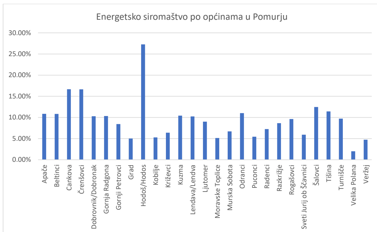
Graf 37: Prikaz udjela kućanstva koja se već suočavaju s energetske siromaštvom po pojedinim općinama u Pomurju
