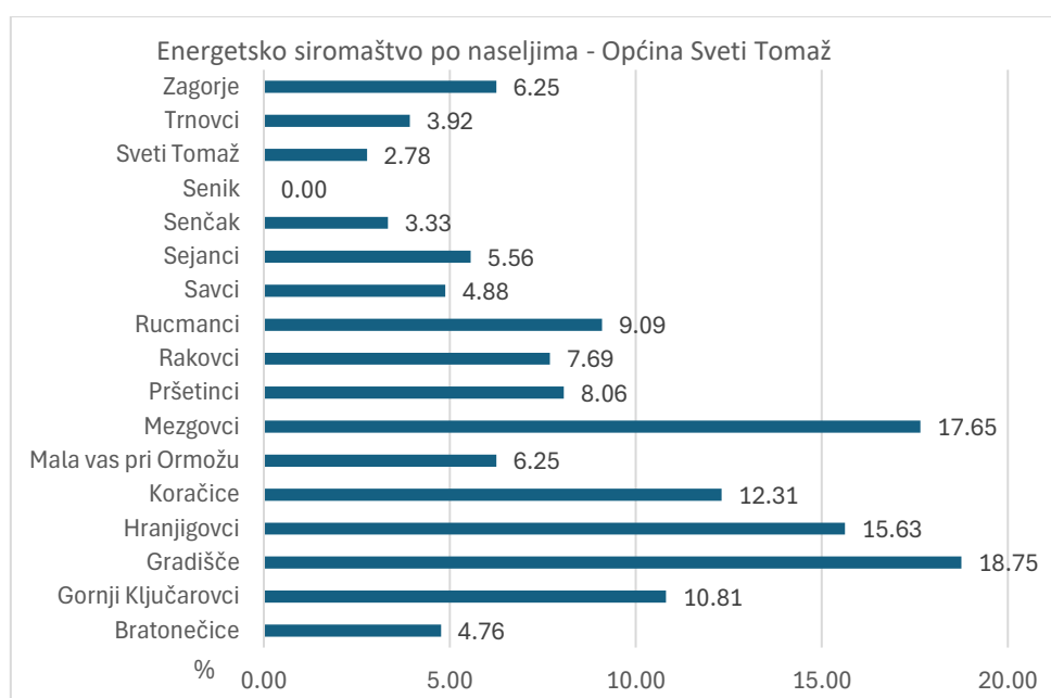
Graf 30: Energetsko siromaštvo po naseljima – Općina Sveti Tomaž
