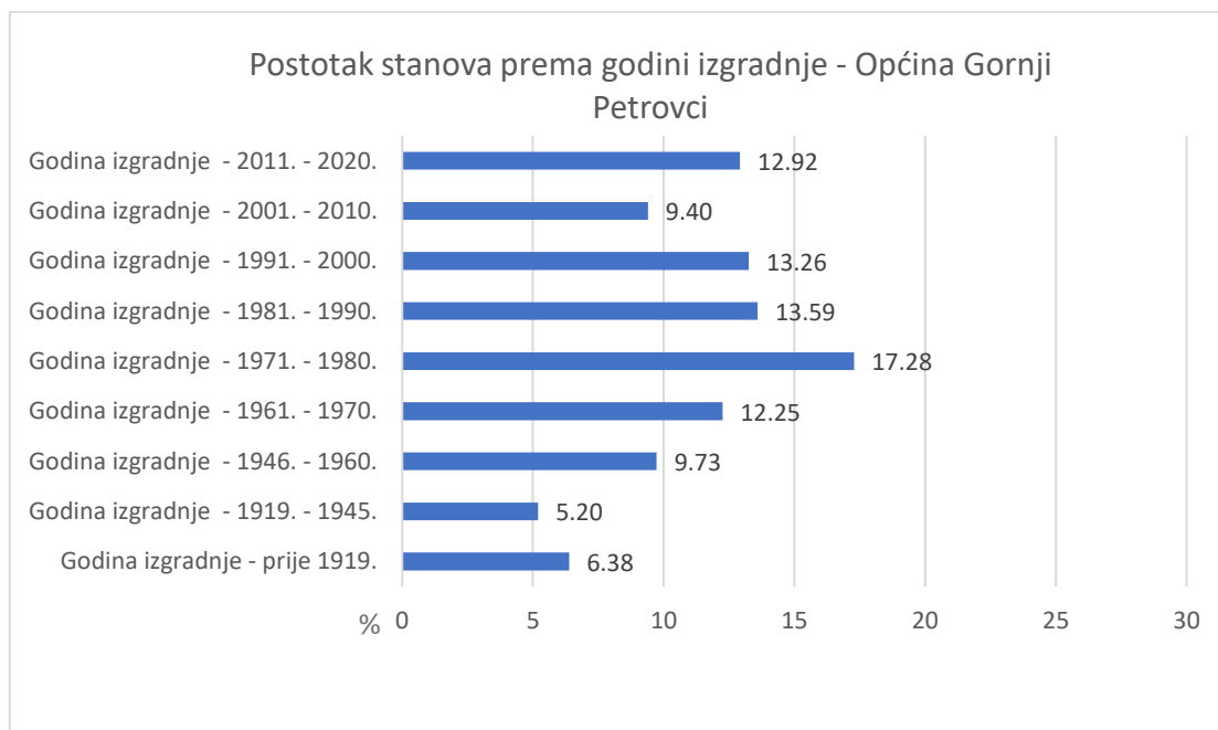
Graf 140: Postotak stanova prema godini izgradnje u Općini Gornji Petrovci (izvor: Statistički ured Republike Slovenije)
