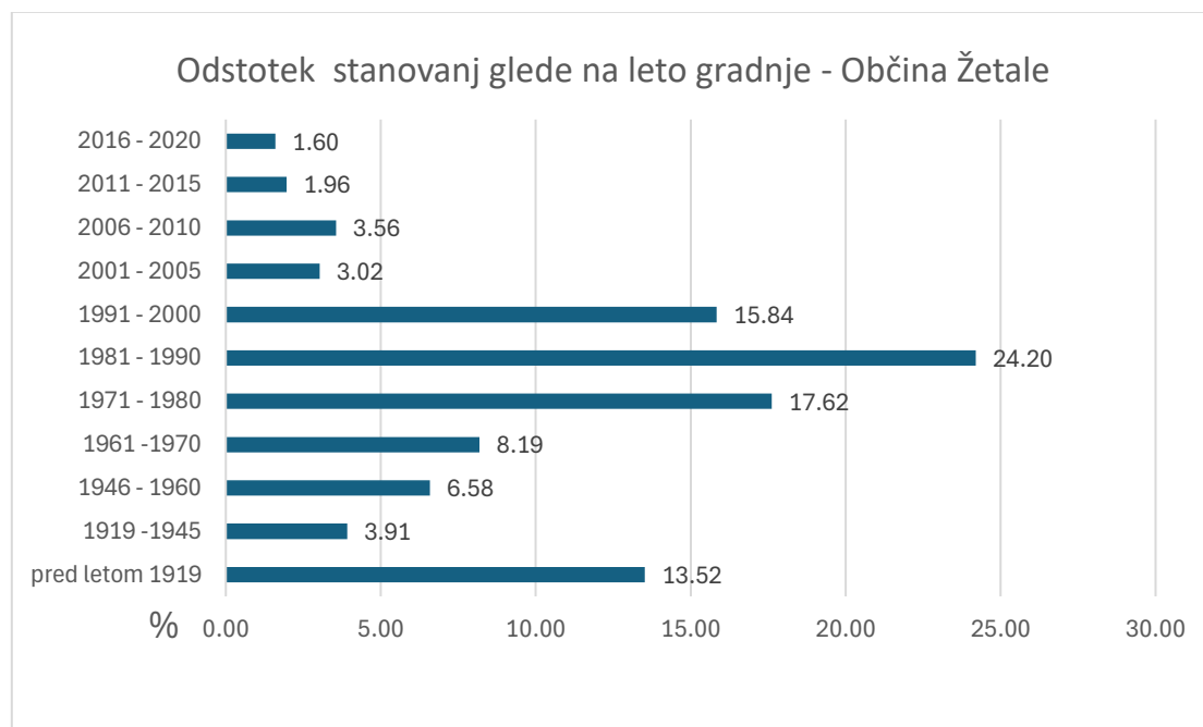
Graf 299: Odstotek stanovanj glede na leto gradnje – Občina Žetale
