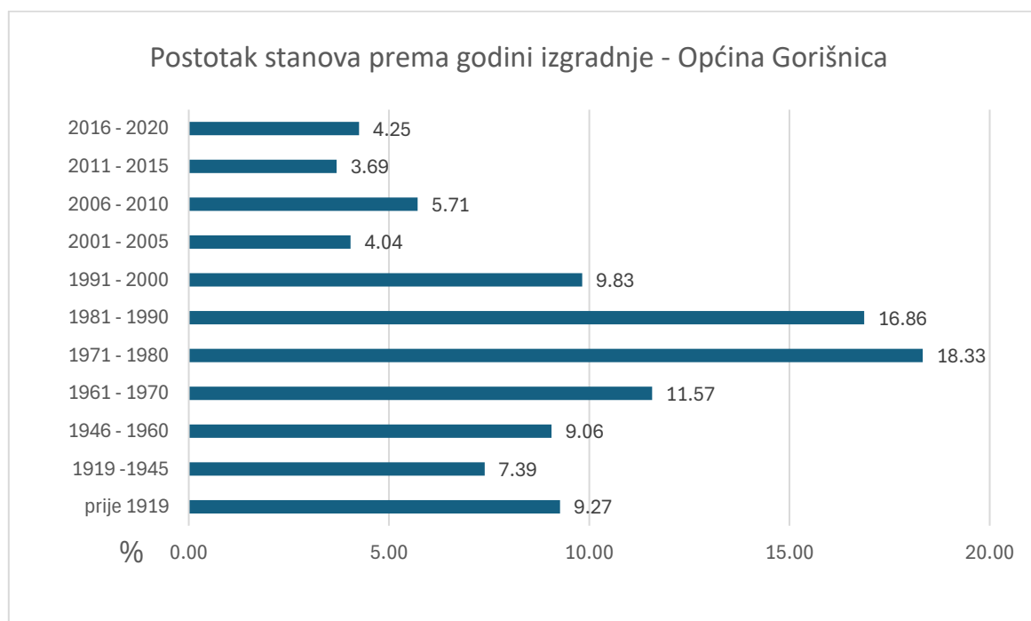
Graf 98: Postotak stanova prema godini izgradnje – Općina Gorišnica
