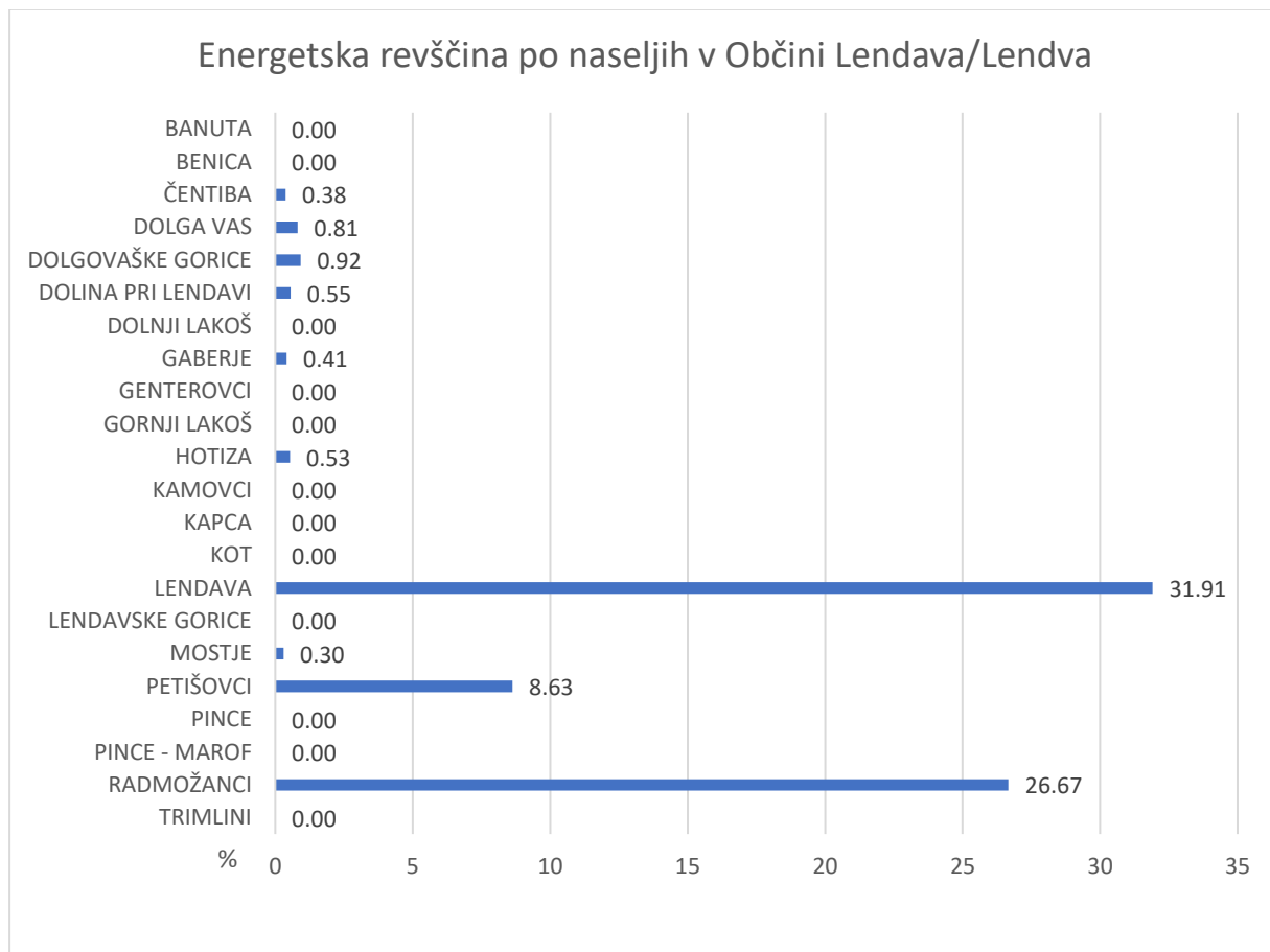
Graf 216: Energetska revščina v odstotkih po naseljih v Občini Lendava/Lendva
