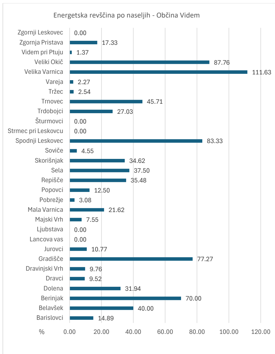
Graf 198: Energetska revščina po naseljih - Občina Videm
