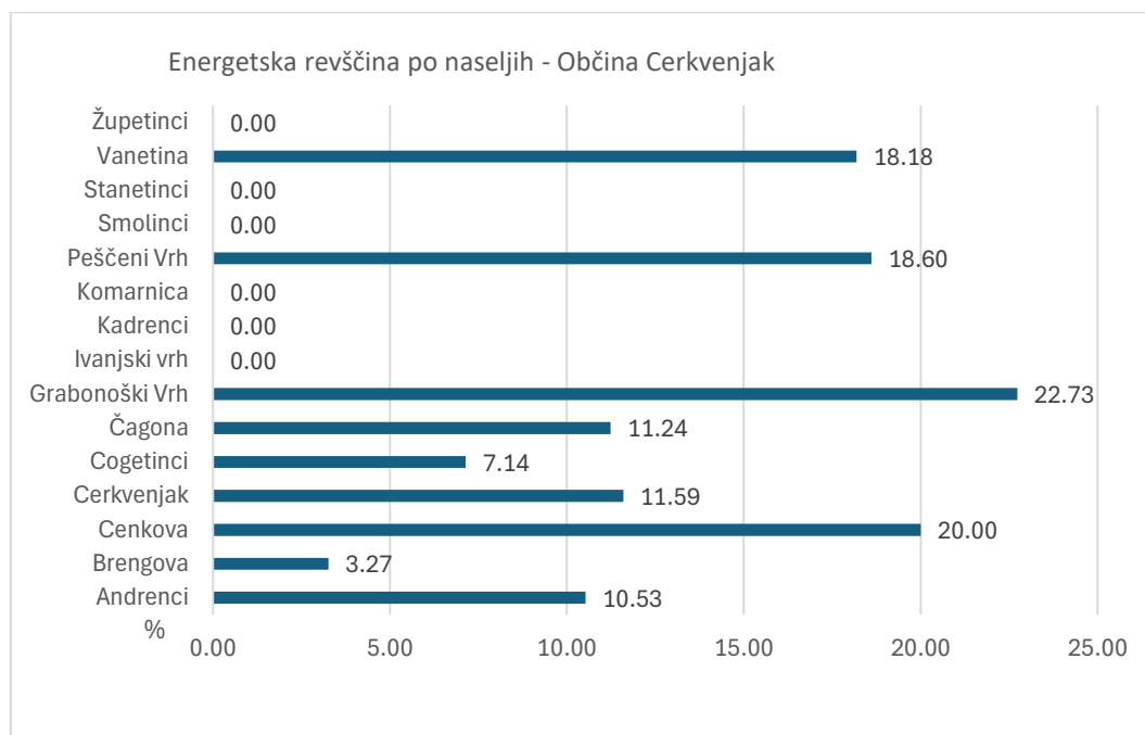
Graf 173: Energetska revščina po naseljih - občina Cerkevjak
