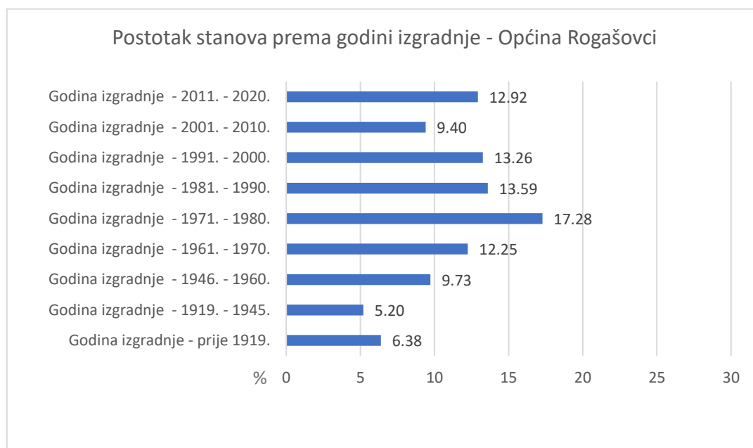
Graf 154: Postotak stanova prema godini izgradnje u Općini Rogašovci (izvor: Statistički ured Republike Slovenije)
